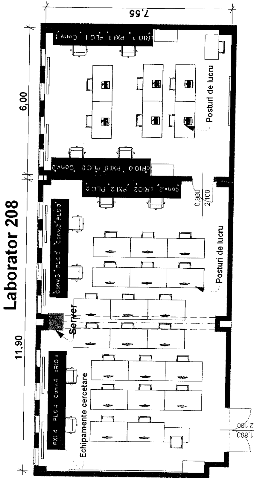
P1 - Planșa de ansamblu – Laborator 208
